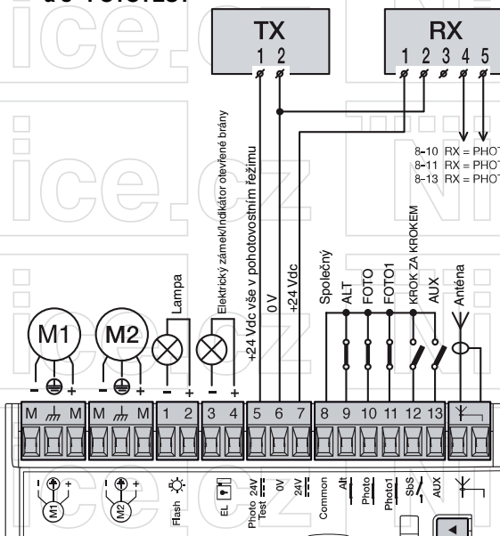
C Zapojení bez "pohotovostního režimu" a s "FOTOTEST"
